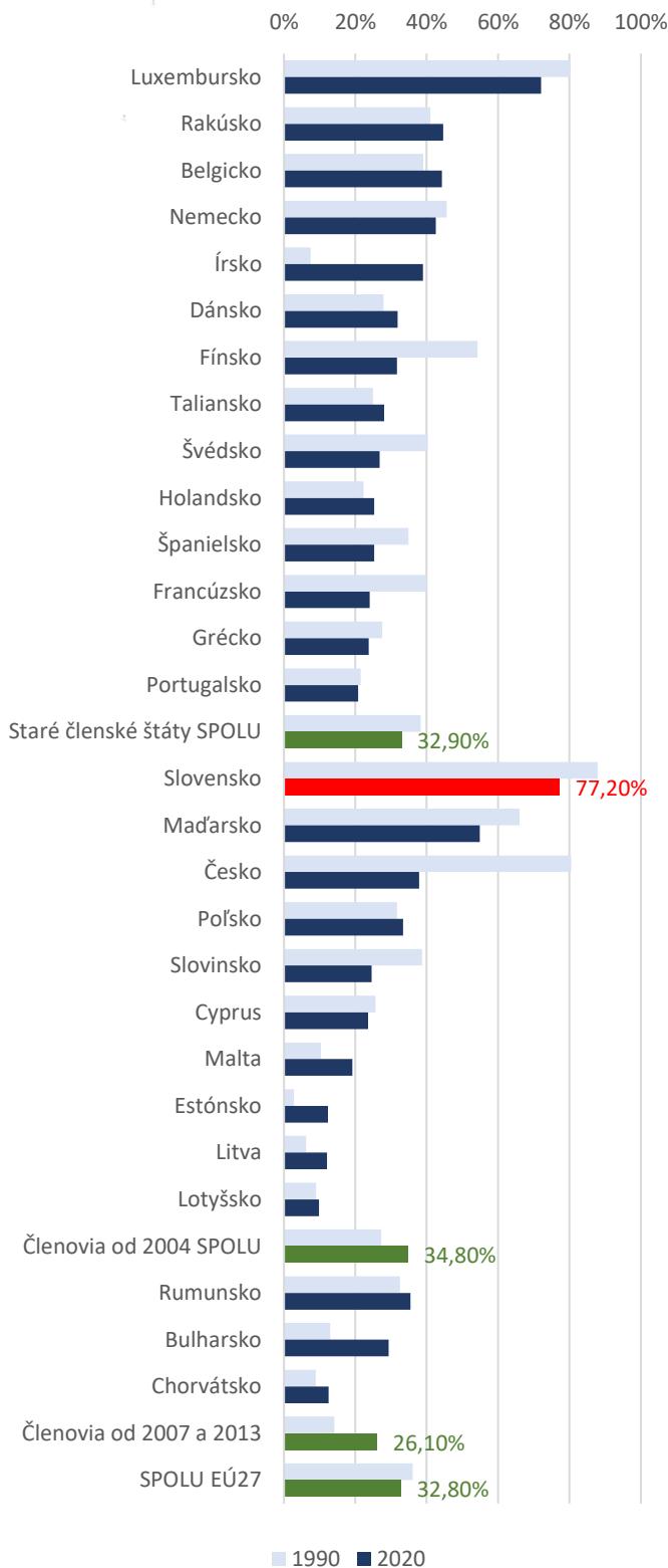
Graf: Podiel imigrantov žijúcich v štátoch dnešnej EÚ27 pochádzajúcich z ostatných krajín dnešnej EÚ27 (v % z celkovej imigrácie do uvedených štátov), pre roky 1990, 2020
